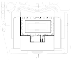
PŮDORYS 3.NP
