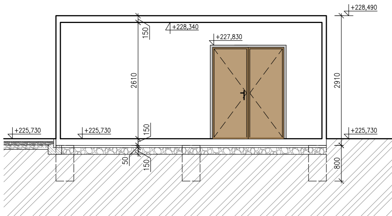
ŘEZ A-A
