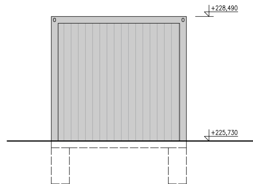
POHLED PŘÍČNÝ
