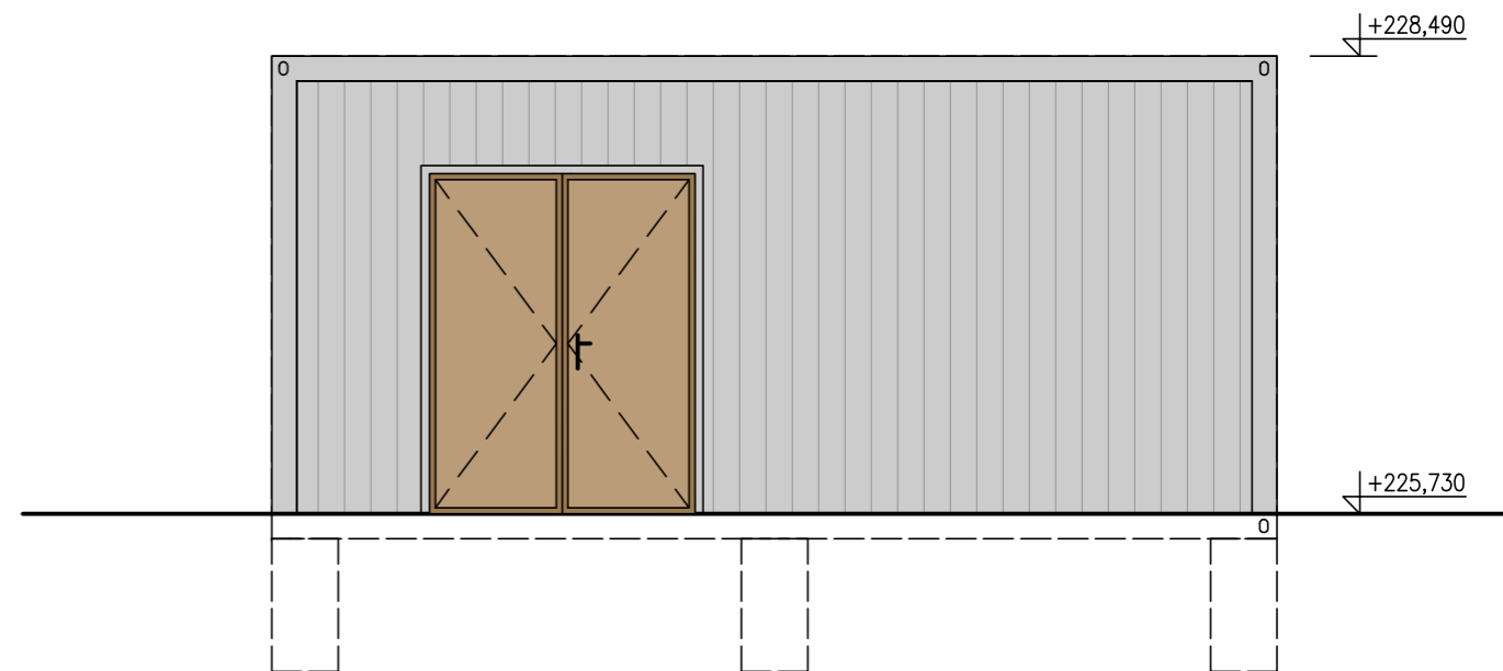
POHLED PŘÍČNÝ
